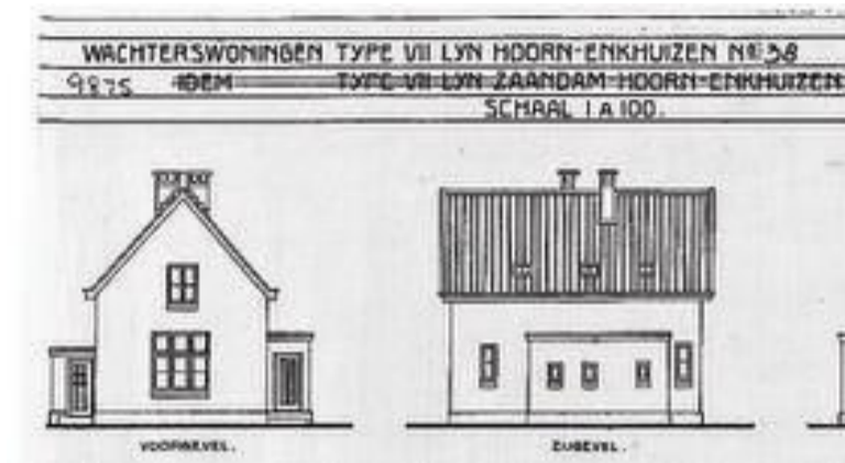
Tekening van het type wachterswoning dat bij Enkhuizen stond. Archief Nederlandse Spoorwegen. ARCHIEF NEDERLANDSE SPOORWEGEN.
